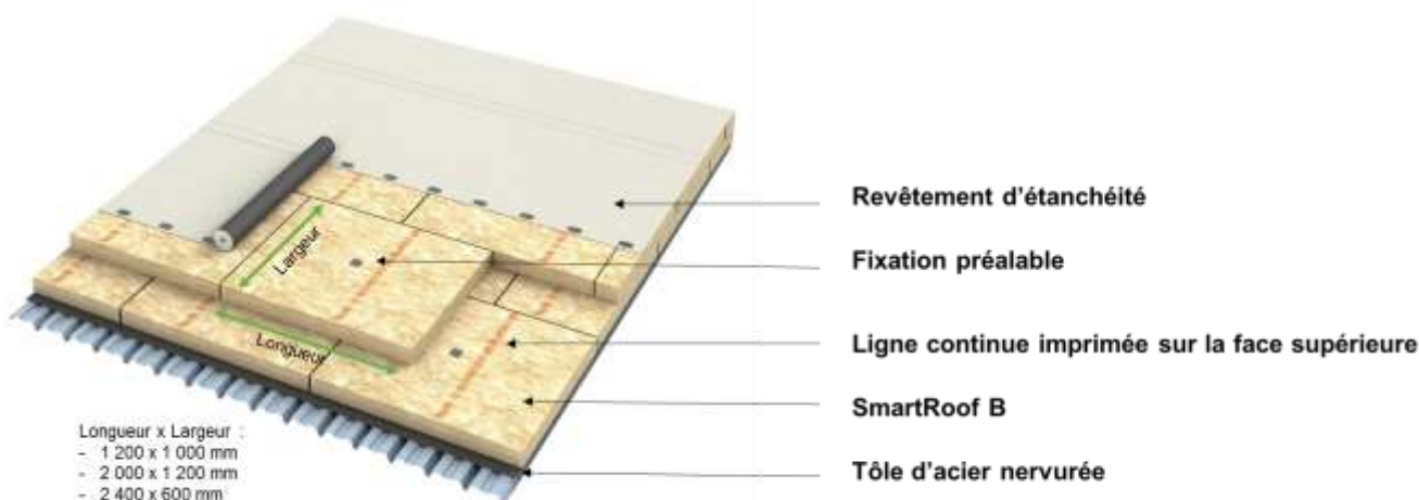
Figure 1 – Sens de pose des panneaux SmartRoof B sur TAN conforme à la norme NF DTU 43.3
