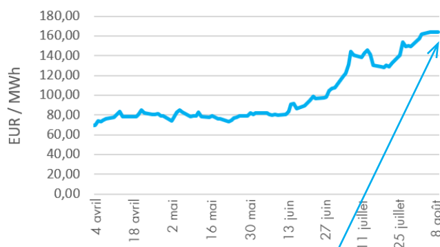
EEX: Gas naturel (Europe centrale), année+1
