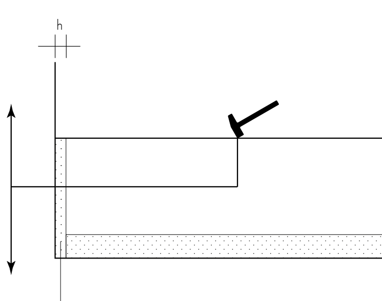
A 3 jelű elem, mint testhangszigetelő réteg követelményei ( d \geq 10 mm, E_d \leq 0,5 MN/m 2 )
